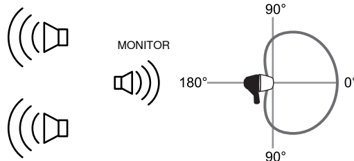
Posizioni consigliate degli altoparlanti per i microfoni cardiode
