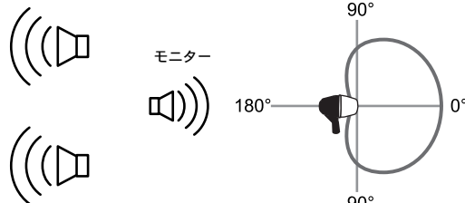
カーディオイドマイクロホン向けスピーカーの推奨配置
