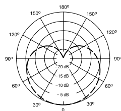
1000 Hz Diagramma polare tipico
