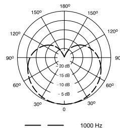
Courbe de directivité typique
