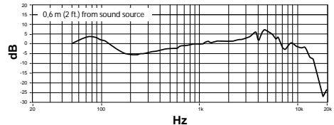
주파수 응답
