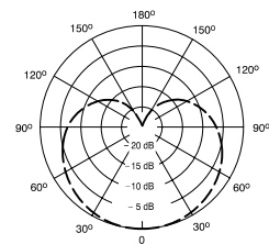
극성 패턴
