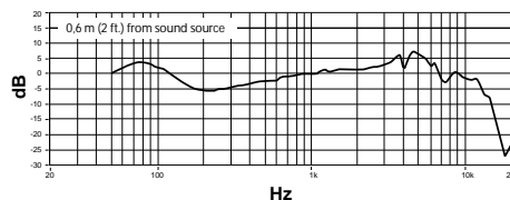
Типичная частотная характеристика
